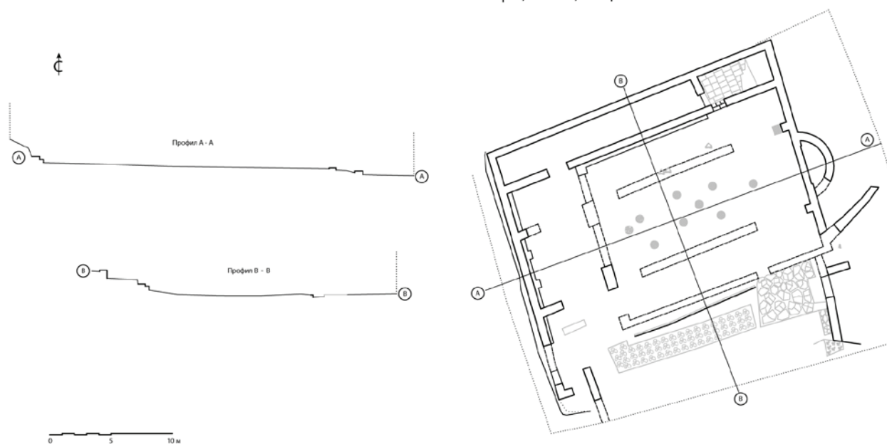
Обр. 1. Ранновизантийска базилика в с. Гела – план.
